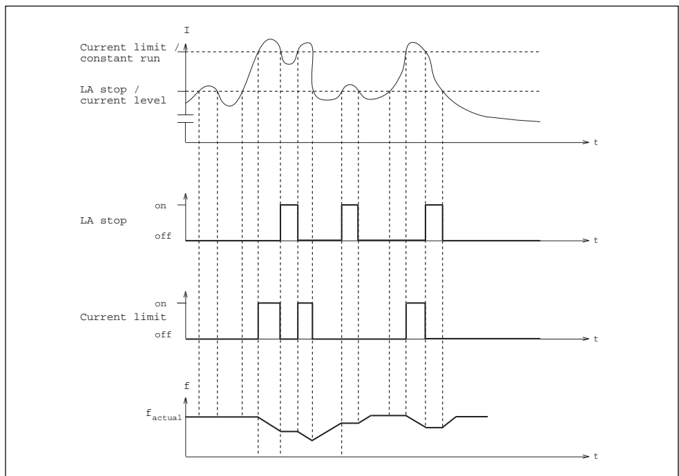
Рис. 62 b Функция LA Стоп и ограничение тока
