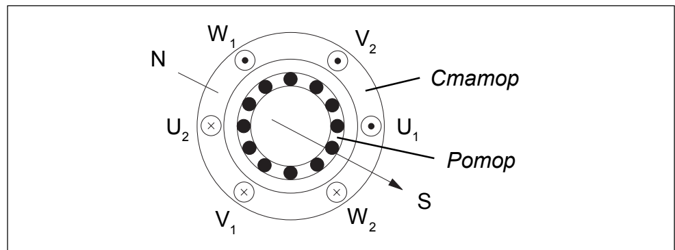
Рис. 1 Схема беличьего колеса
