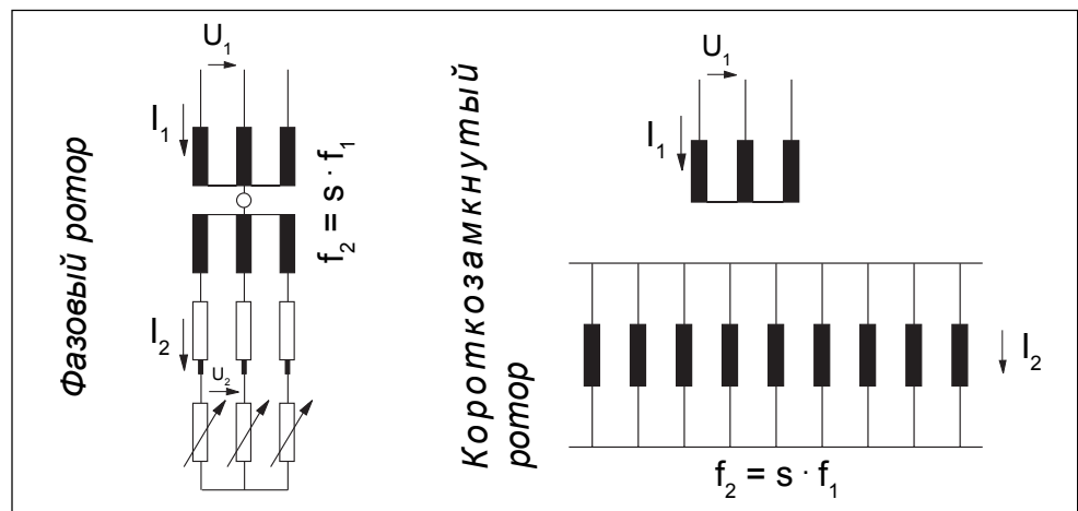
Рис. 2 Сравнение фазового ротора с короткозамкнутым ротором
