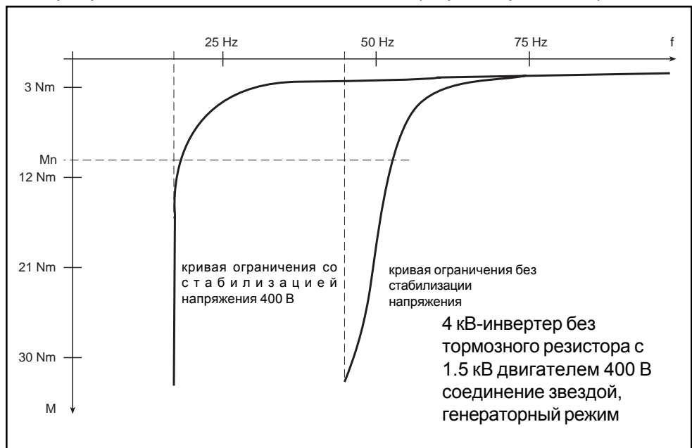
Рис. 50 Типичные кривые ограничения для ОР-ошибки в генераторном режиме
