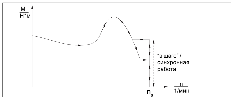
Рис. 16 Моментно- скоростная характеристика реактивного синхронного двигателя
